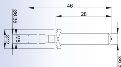
Reichner Indenter 0.2 R 120^\circ
